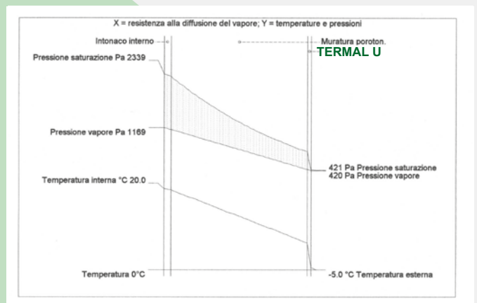
diagramma di Glaser
