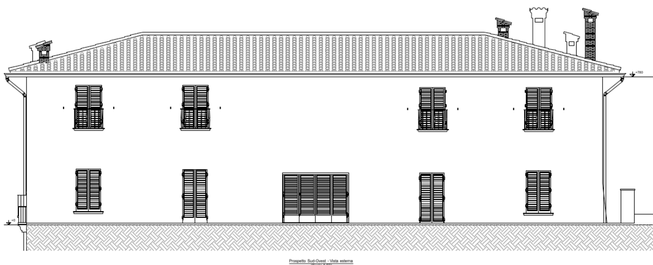
Figura 1 - Prospetto frontale dell'edificio
