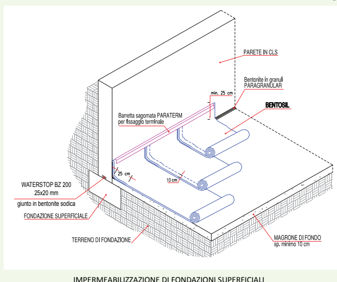
IMPERMEABILIZZAZIONE DI FONDAZIONI SUPERFICIALI
