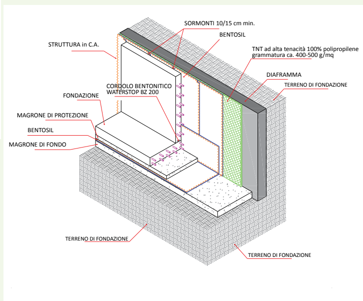
IMPERMEABILIZZAZIONE DI PLATEA E DIAFRAMMA IN C.A.
