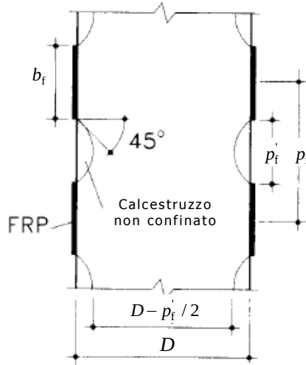
Figura 4-12 – Confinamento discontinuo su una sezione circolare confinata di diametro D : sezione verticale diametrale.
