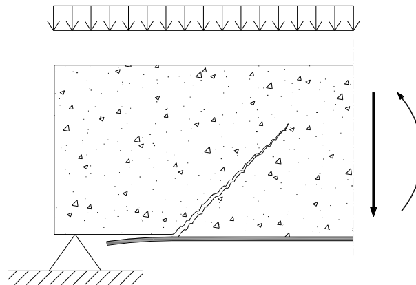
Figura 10-4 – Distacco causato da fessure diagonali da taglio.
