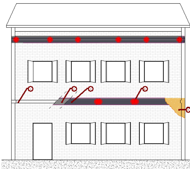
PROSPETTO FRONTALE
