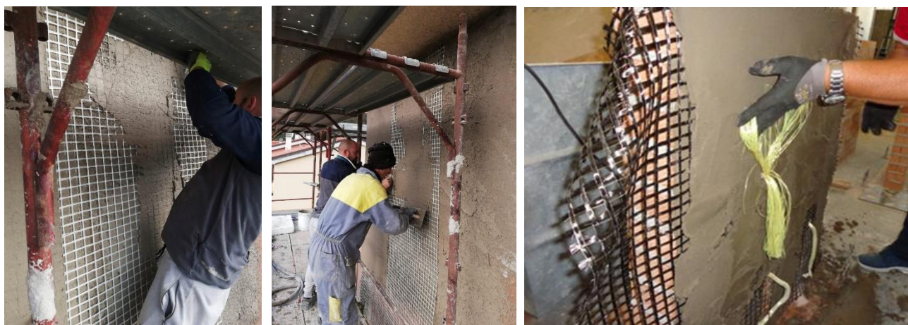
Immagine 14: Rinforzo muratura con FRCM.
