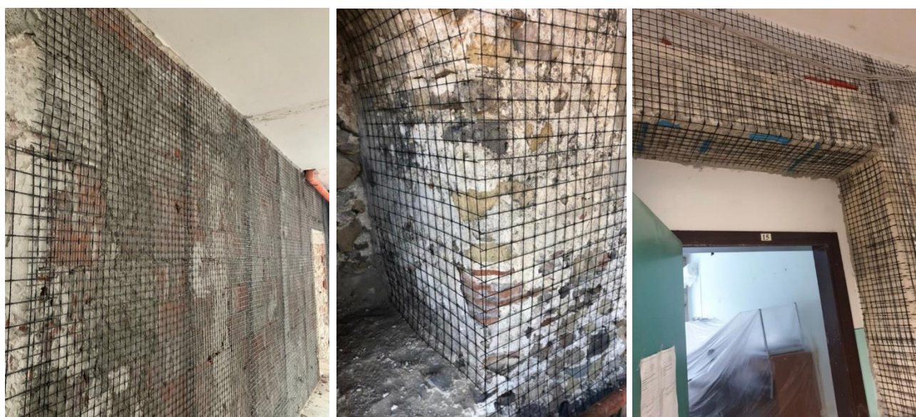
Immagine 17: Applicazioni reti CRM.
