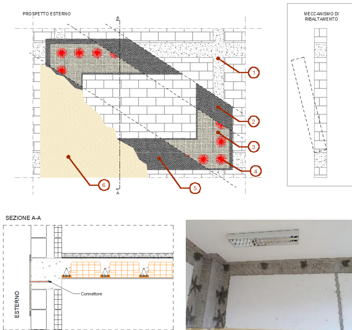
Immagine 9: Sistema antiribalta perimetrale.
